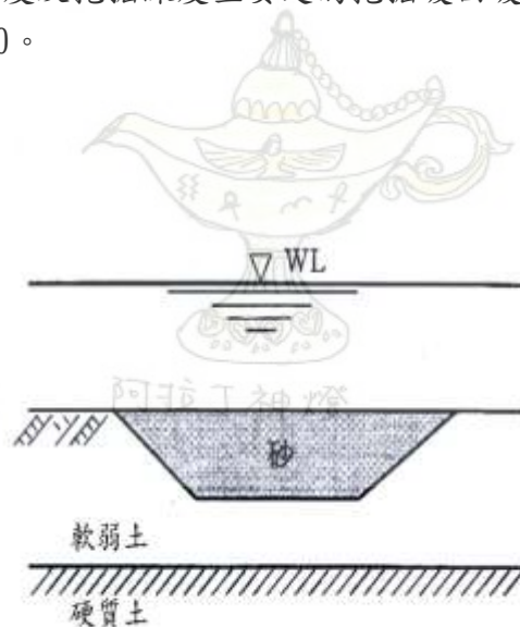
(b) 部份挖掘換置法
