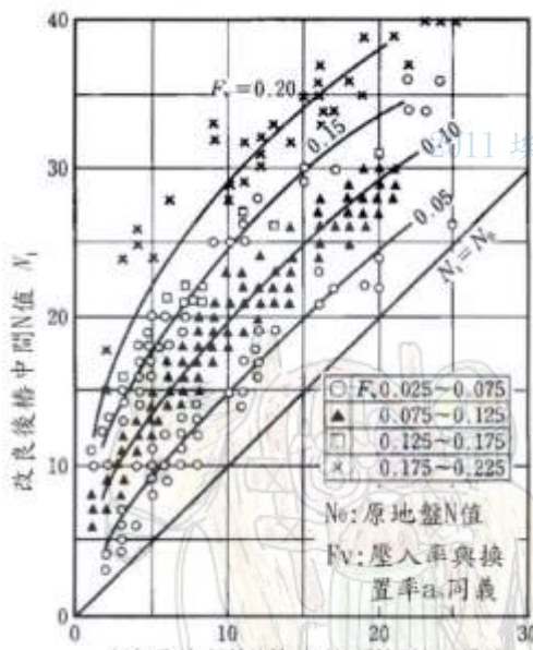
(a) 原地盤 N_0 與樁間 N_1 值的關係
