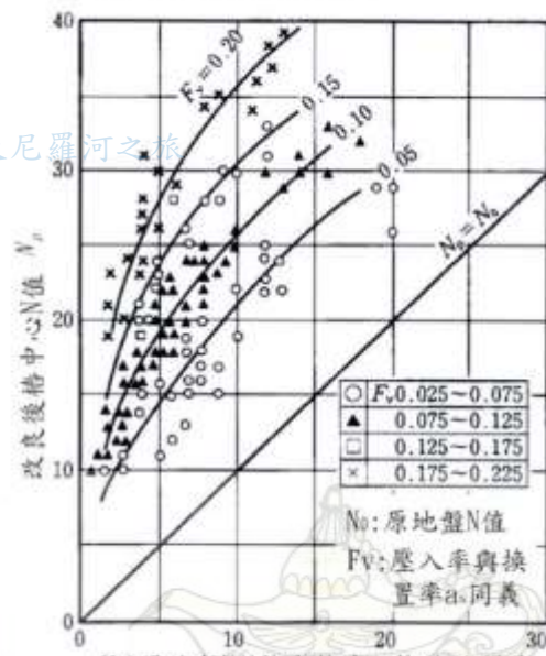
(b) 原地盤 N_0 與樁中心 N_p 值的關係
