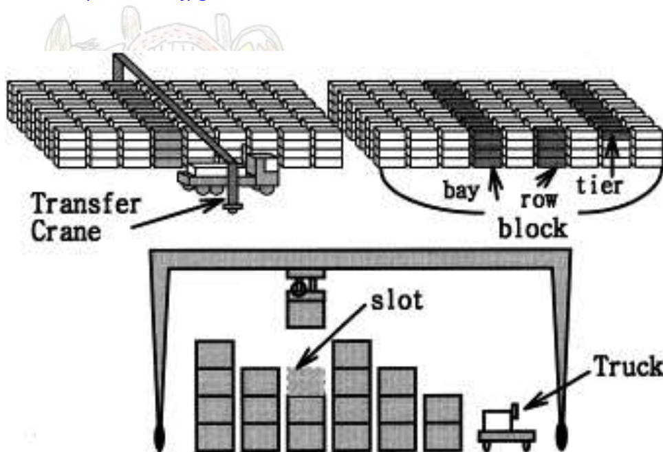
移載機操作示意圖
